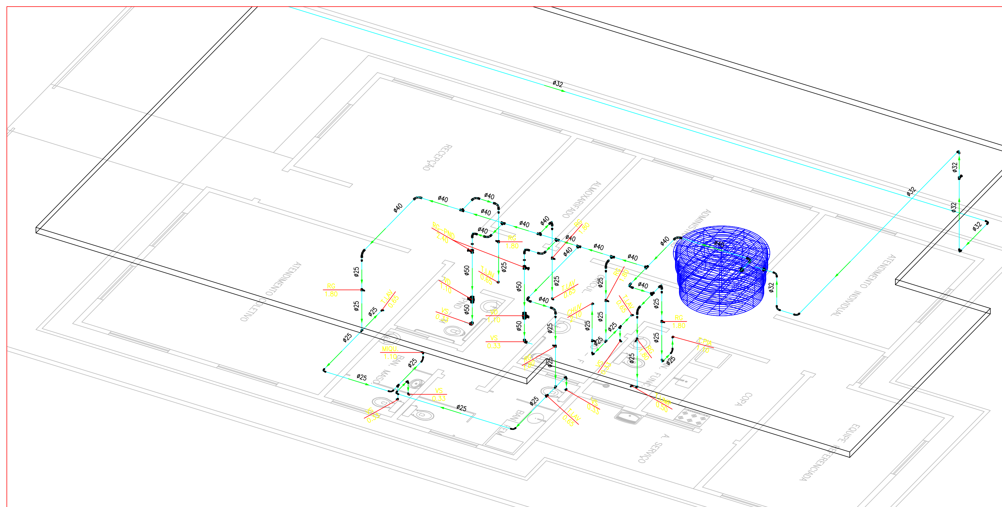
2 DETALHE UNIFILAR EM VISTA ISOMÉTRICA SEM ESCALA
