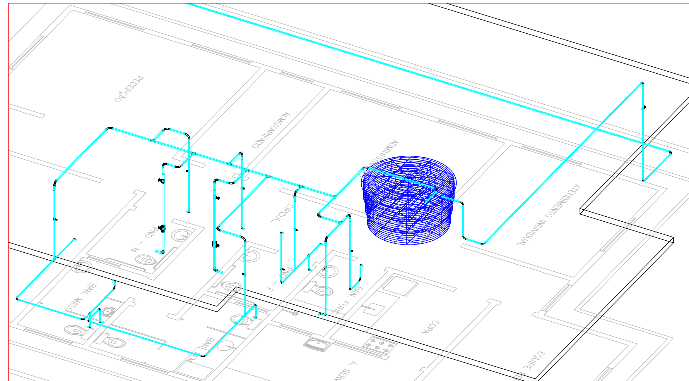
3 DETALHE 3D EM VISTA ISOMÉTRICA SEM ESCALA
